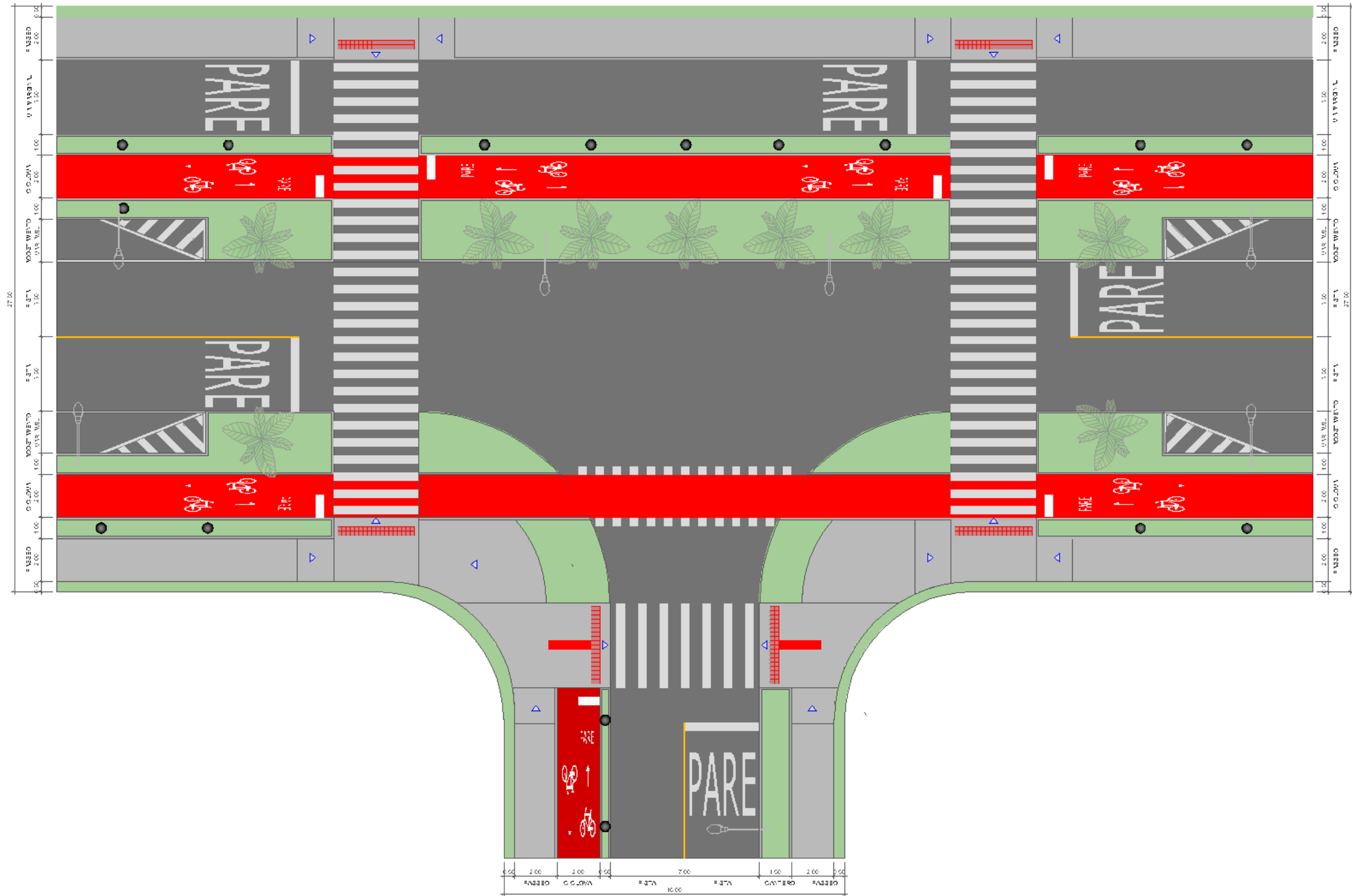
Figura 75 - Boulevard Estrada da Ilha 31 m x Vias 16 m
