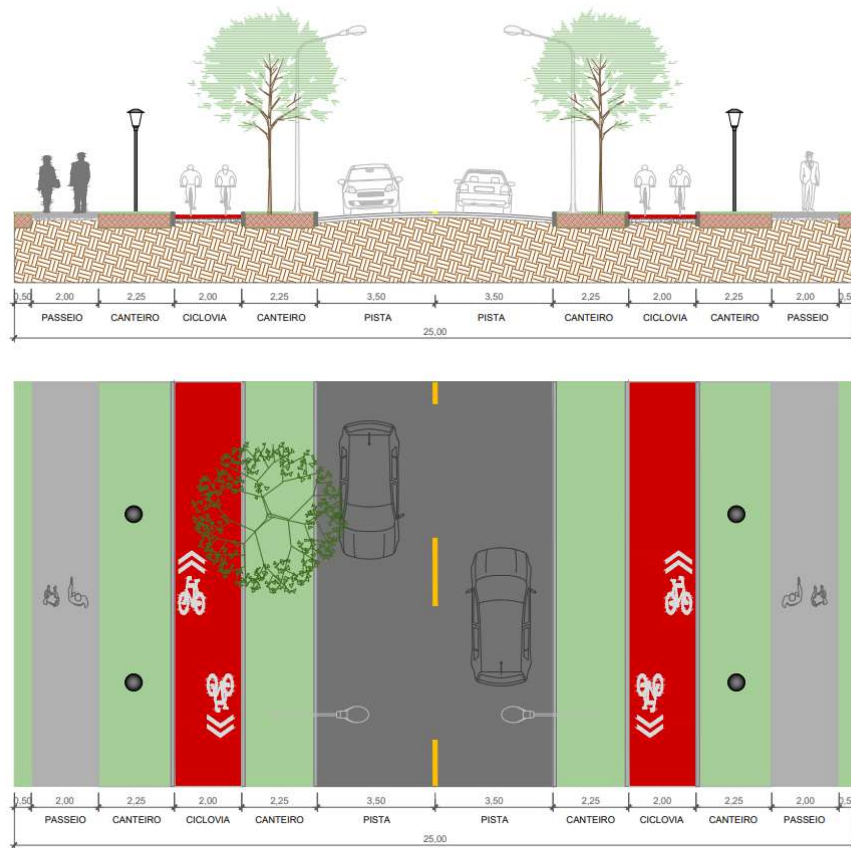
Figura 68 - Boulevard Vale Verde - Seção de 25 m
