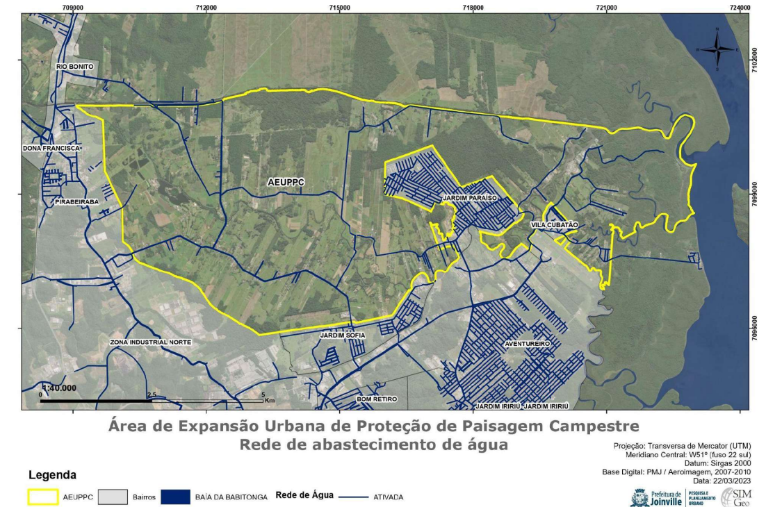
Figura 21 - Rede de abastecimento de água
