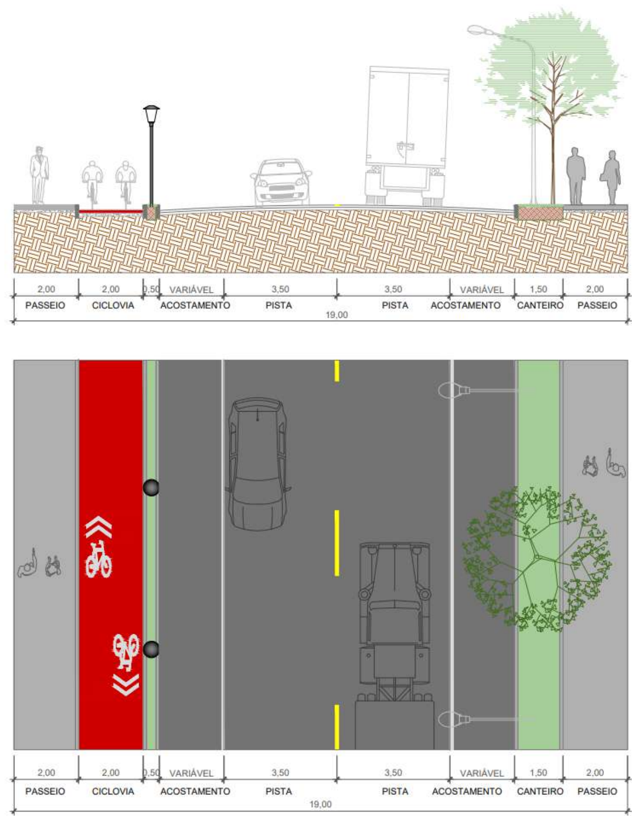
Figura 65 - Boulevard Estrada da Ilha - Seção de 19 m
