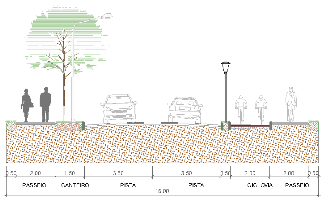
Figura 71 - Vias - Seção de 16 m
