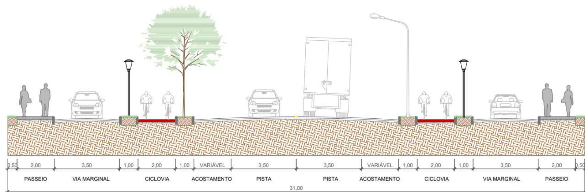
Figura 66 - Boulevard Estrada da Ilha - Seção de 31 m
