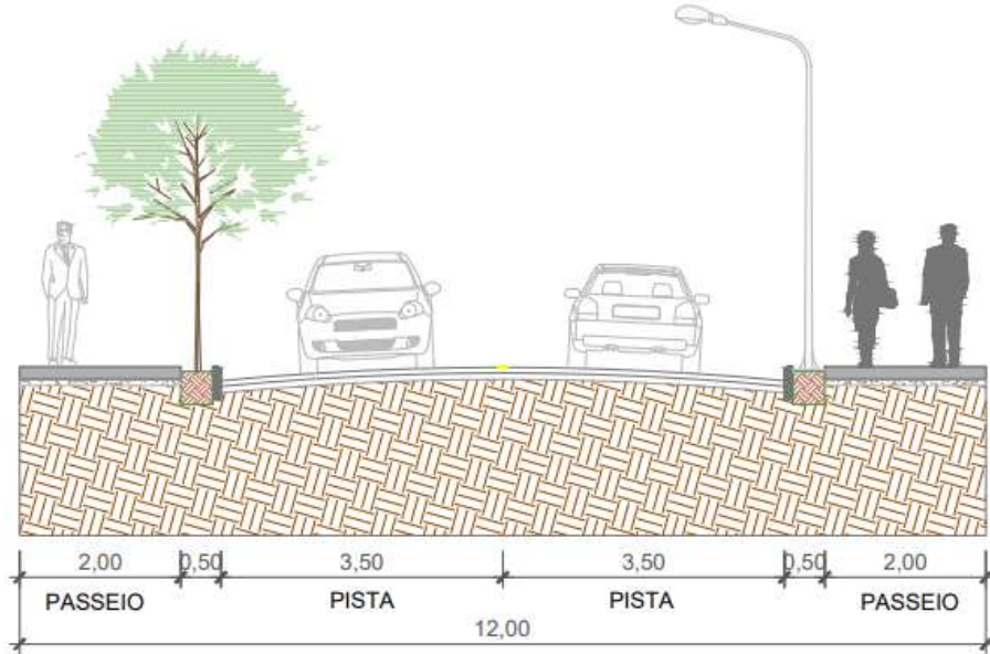
Figura 72 - Vias - Seção de 12 m
