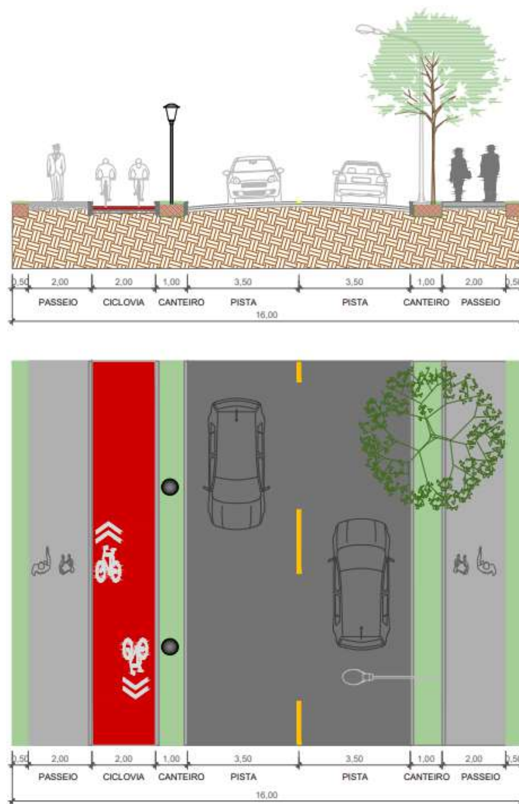
Figura 67 - Boulevard Vale Verde - Seção de 16 m
