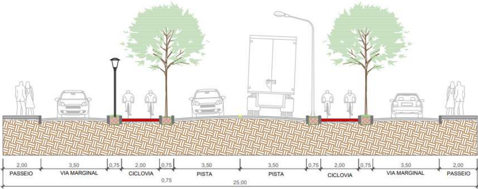
Figura 69 - Boulevard Cubatão - Seção de 25 m
