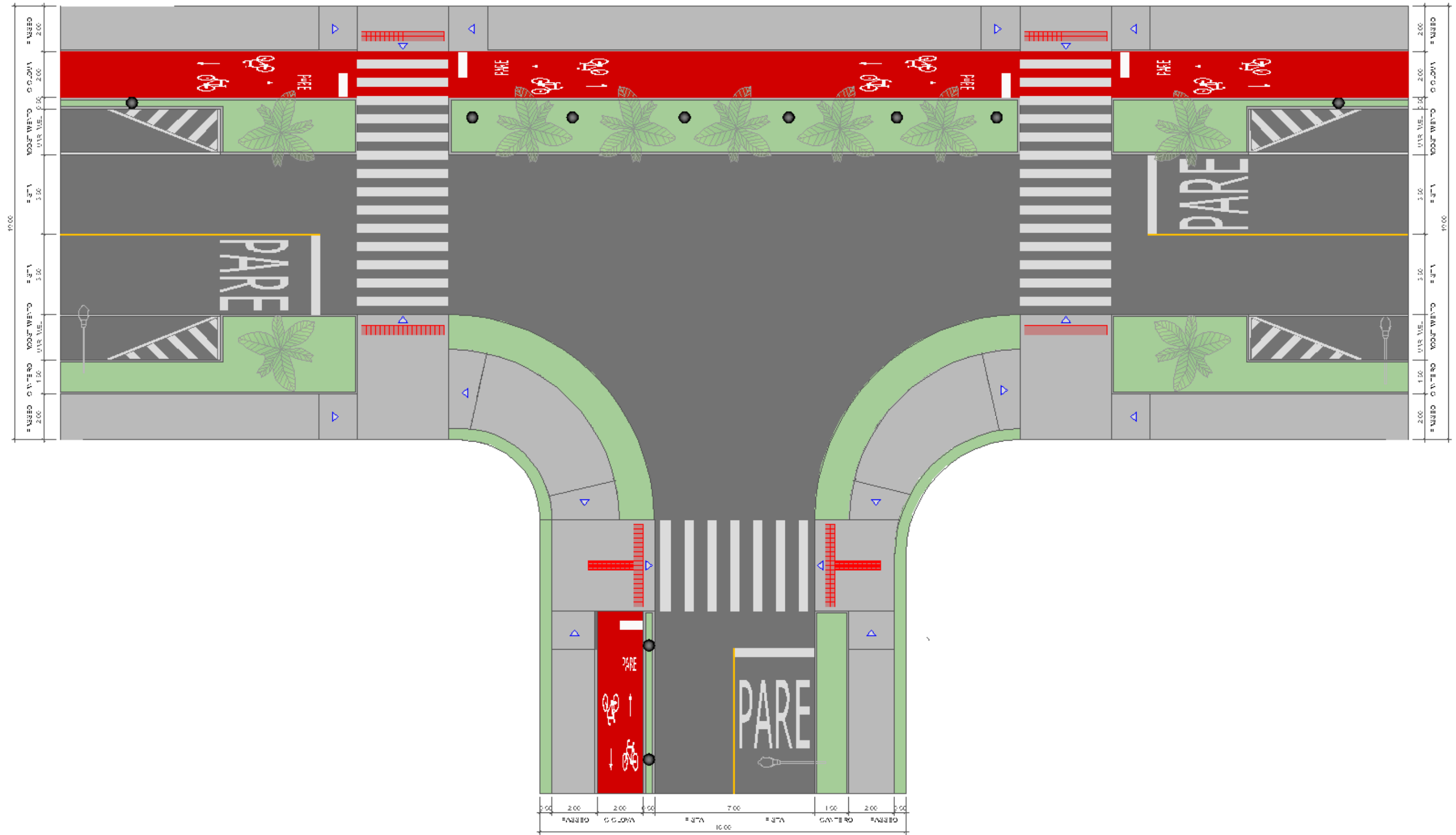
Figura 74 - Boulevard Estrada da Ilha 19 m x Vias 16 m
