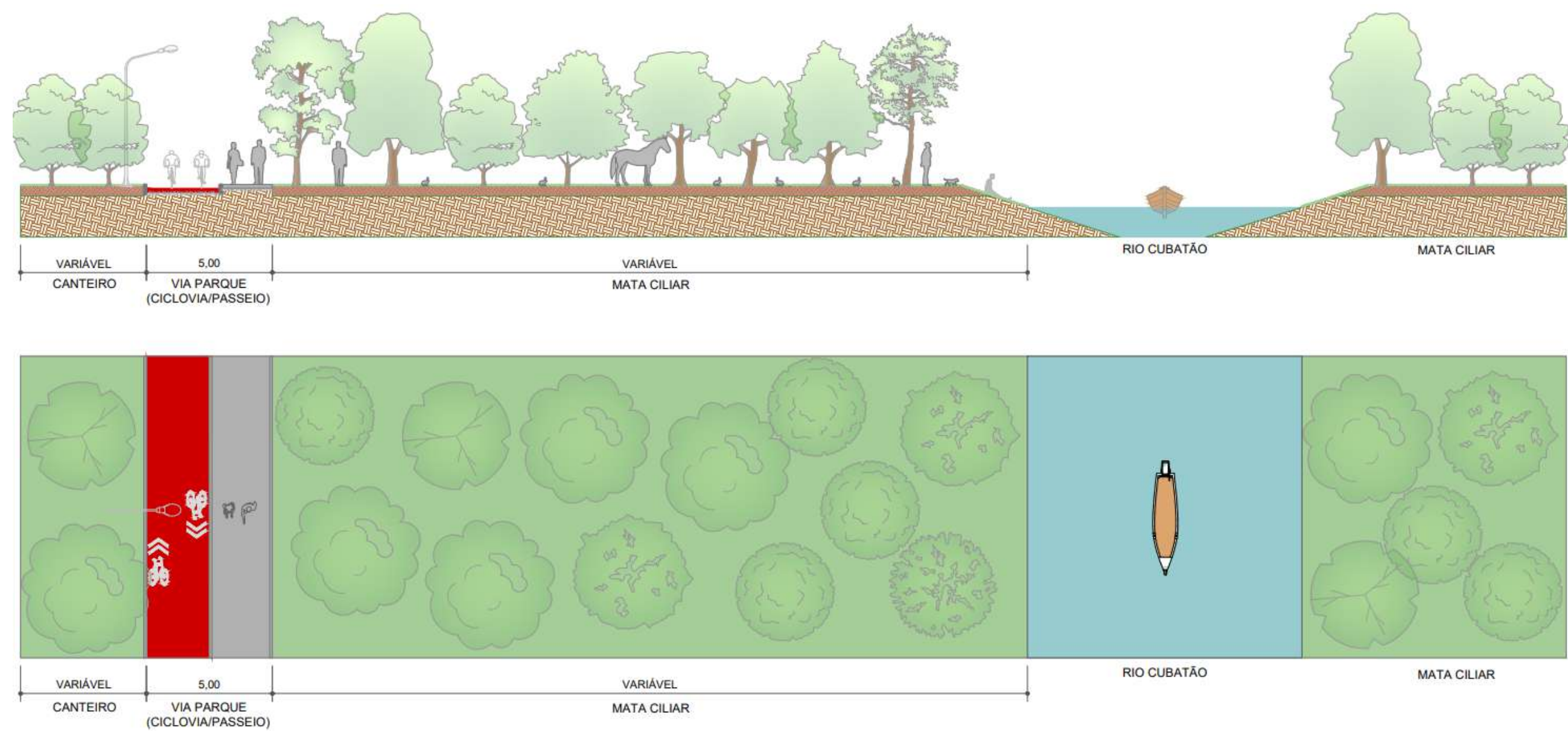
Figura 70 - Via Parque Cubatão
